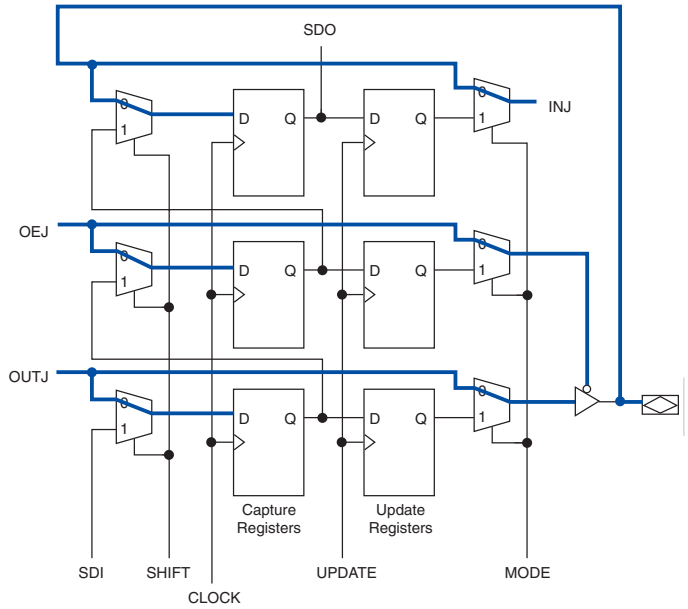
Figure 13. IEEE Std. 1149.1 BST SAMPLE/PRELOAD Mode
